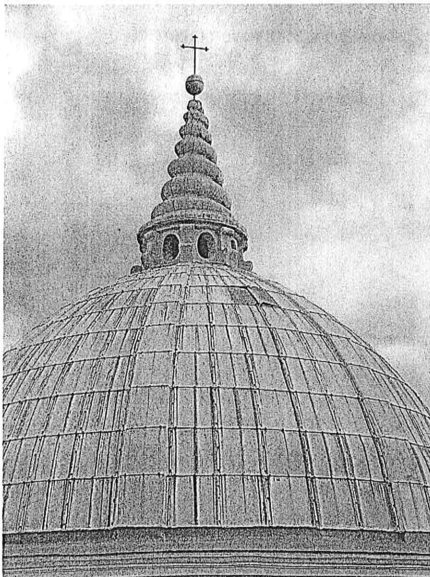
FIG.2 La cupola della chiesa di Santa Brigida vista dai terrazzi prospicienti la cupola della Galleria Umberto I. Si può osservare il distacco della lastra al quarto registro del manto di copertura della cupola in lastre di piombo
